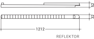
REFLEKTOR
